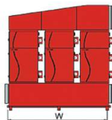
ODF6000 s bočným výpustom, bez ventilátora
